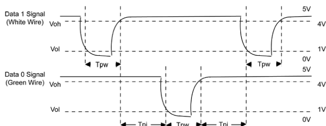
Рис.1: Диаграмма последовательности
