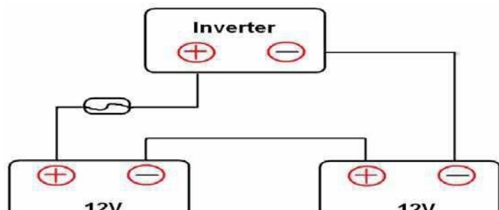
Схема підключення акумулятора 24В постійного струму
