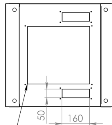
ВИД СВЕРХУ
